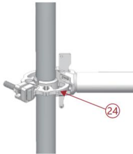
24. Rosette Wedge Coupler
